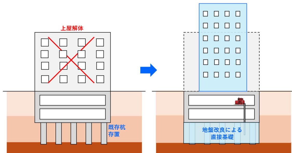
図3 エコタイト-Sによる直接基礎の適用イメージ
