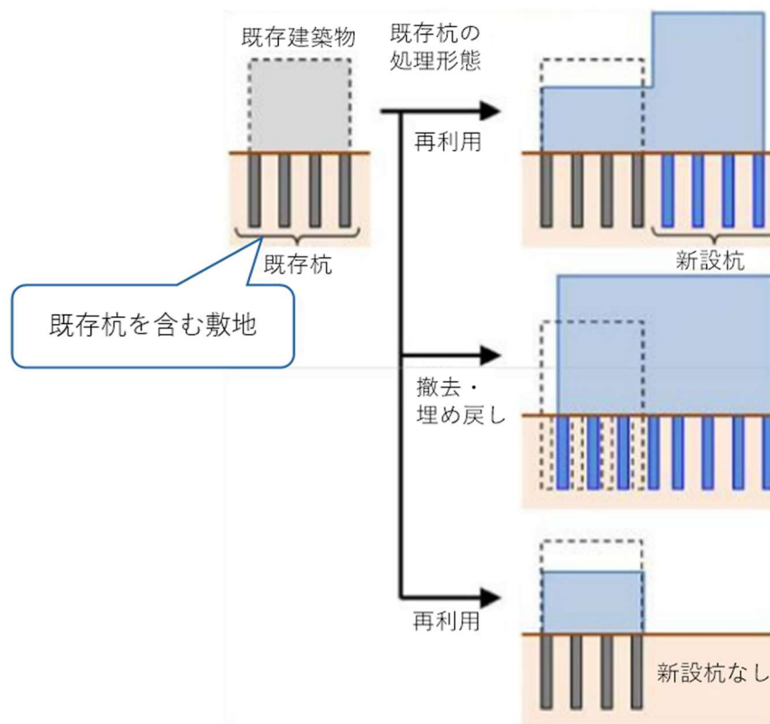
図1 既存杭の扱いイメージ 1)
