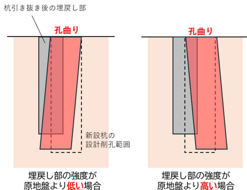
図2 埋戻し部が新設杭に与える施工上の影響の例
